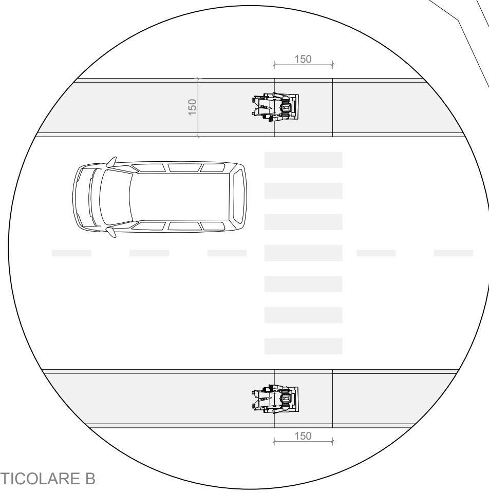
PARTICOLARE B SCALA 1:100
