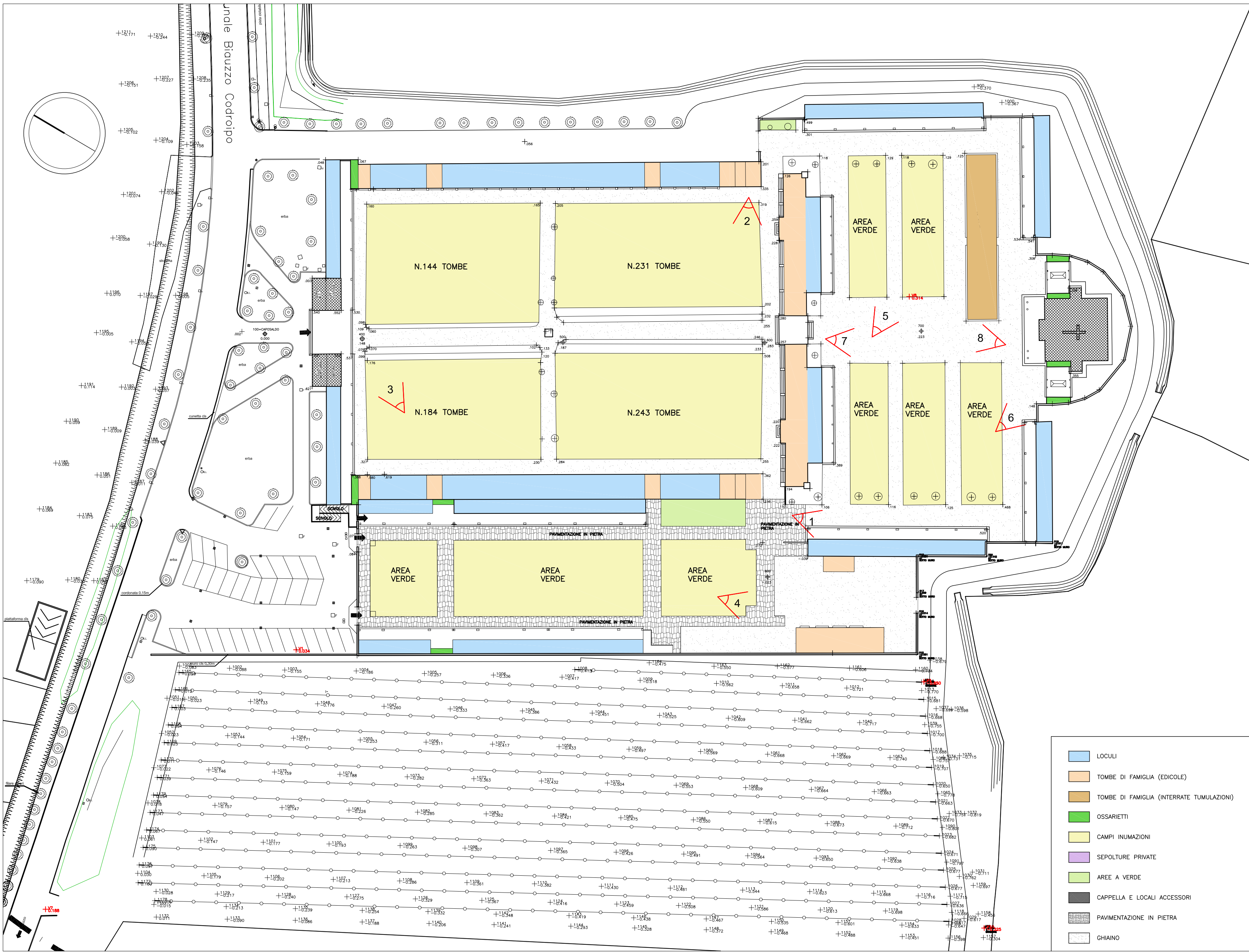
RILIEVO DELLO STATO DI FATTO Scala 1:500
