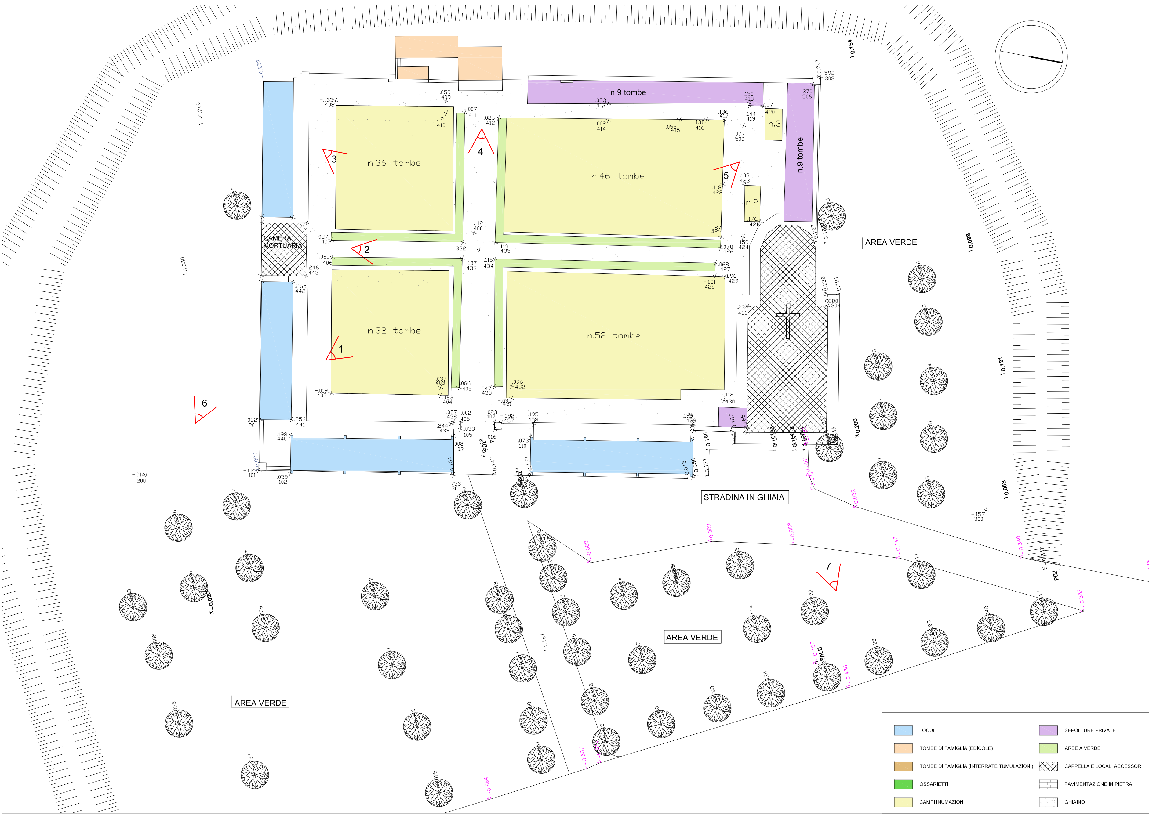
RILIEVO DELLO STATO DI FATTO Scala 1:200
